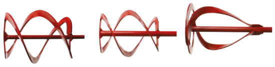
P-02347 <10kg 500W 600min -1 P-02353 <15kg 700W 500min -1 P-22012 <30kg 950W 500min -1
